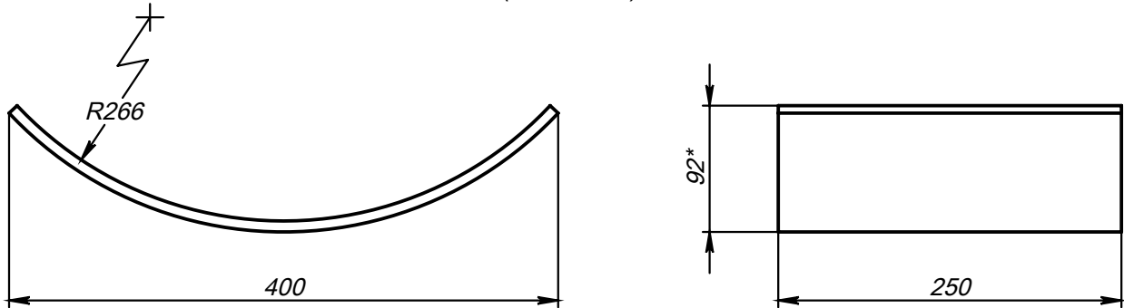
Поз.3 (Ложмент)
